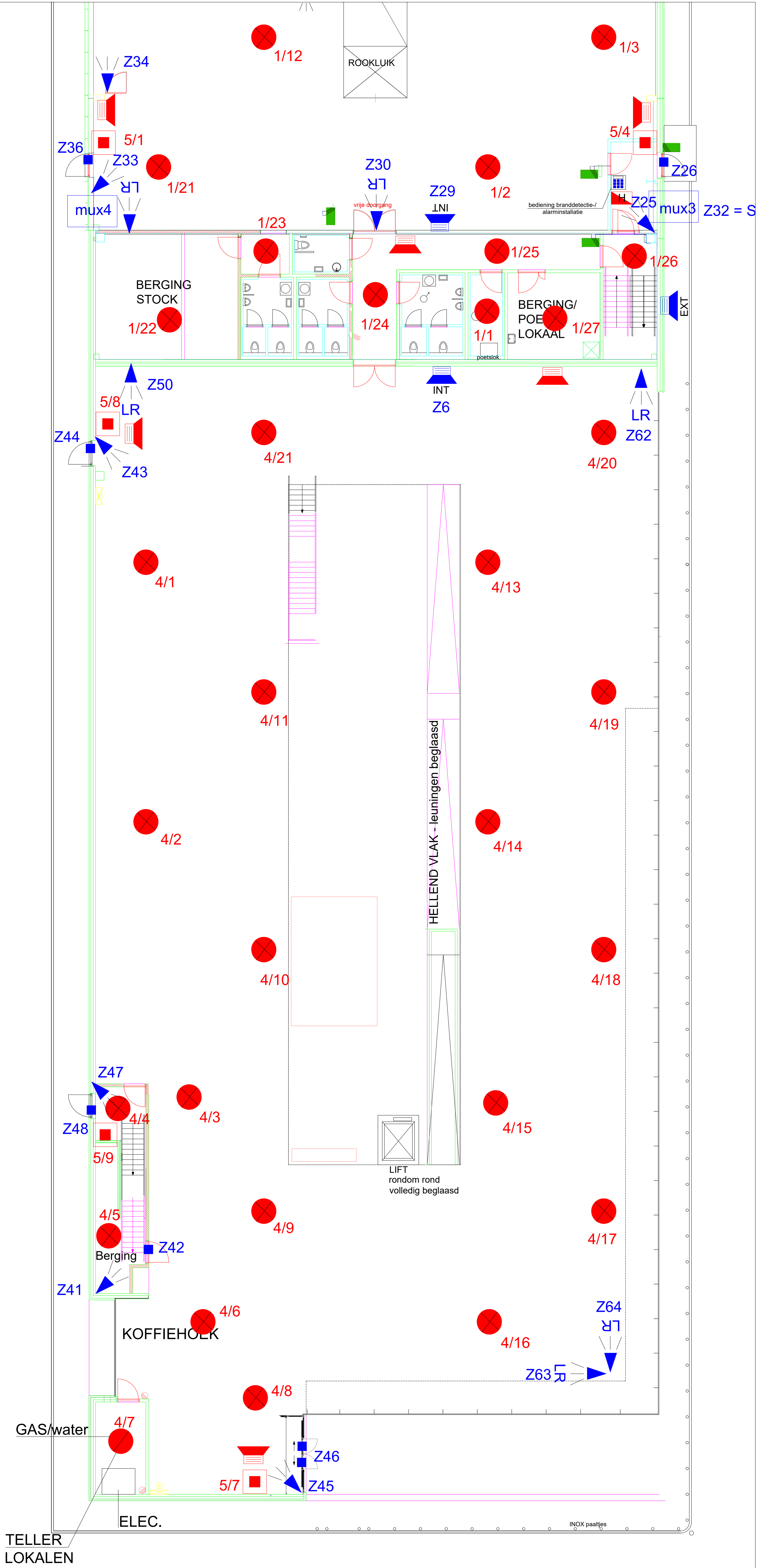
GRONDPLAN SHOWROOM schaal 1/100
