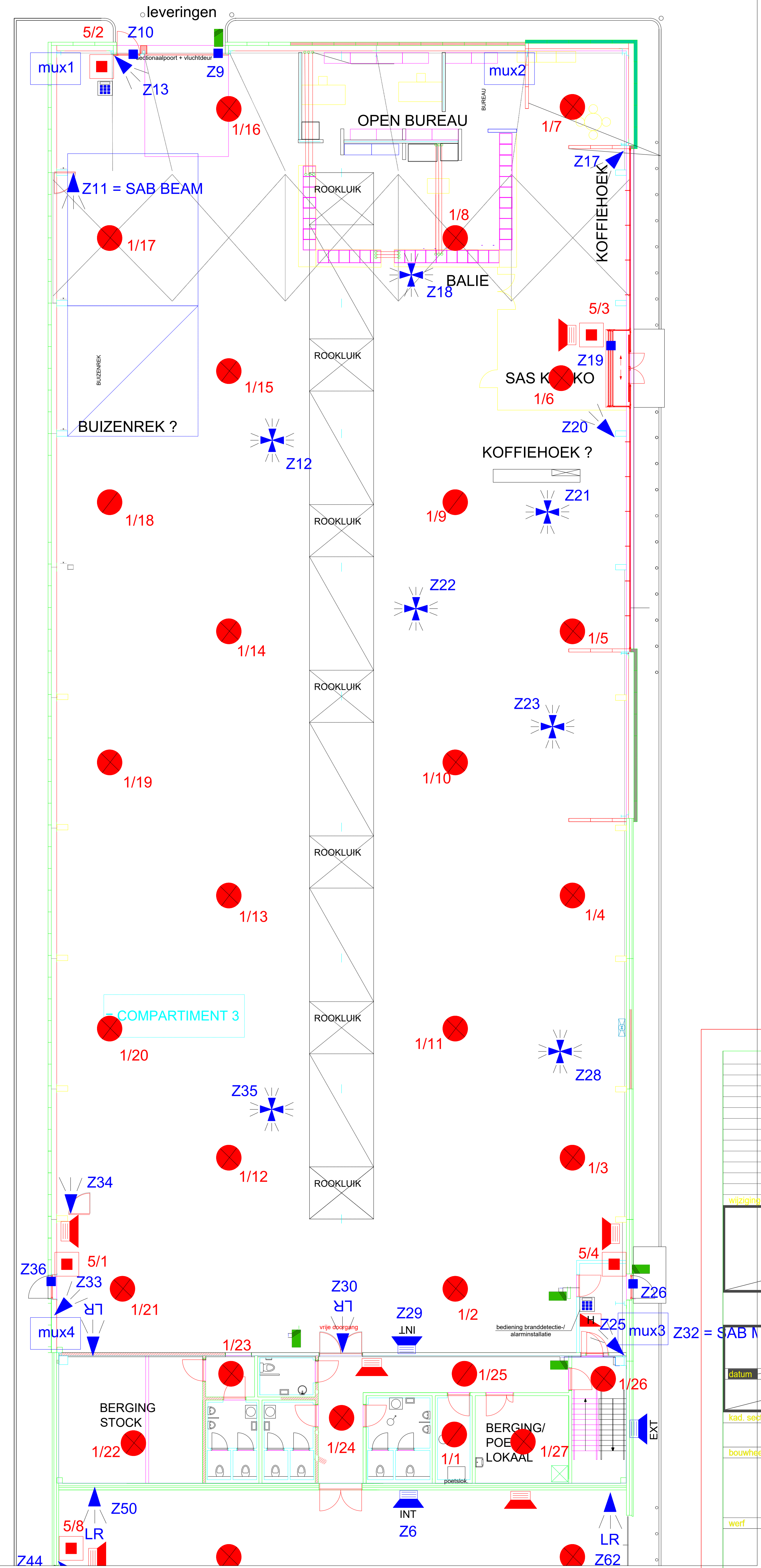
GRONDPLAN SANICENTER schaal 1/100
